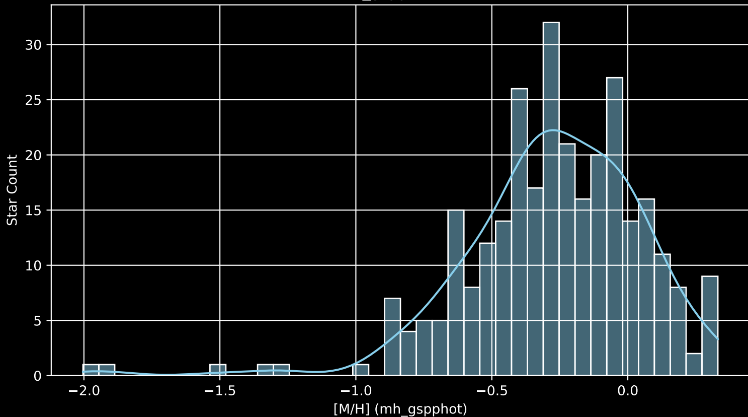
GALAH DR4 Field: [150] [M/H] (mh_gspphot) (n= 295)
