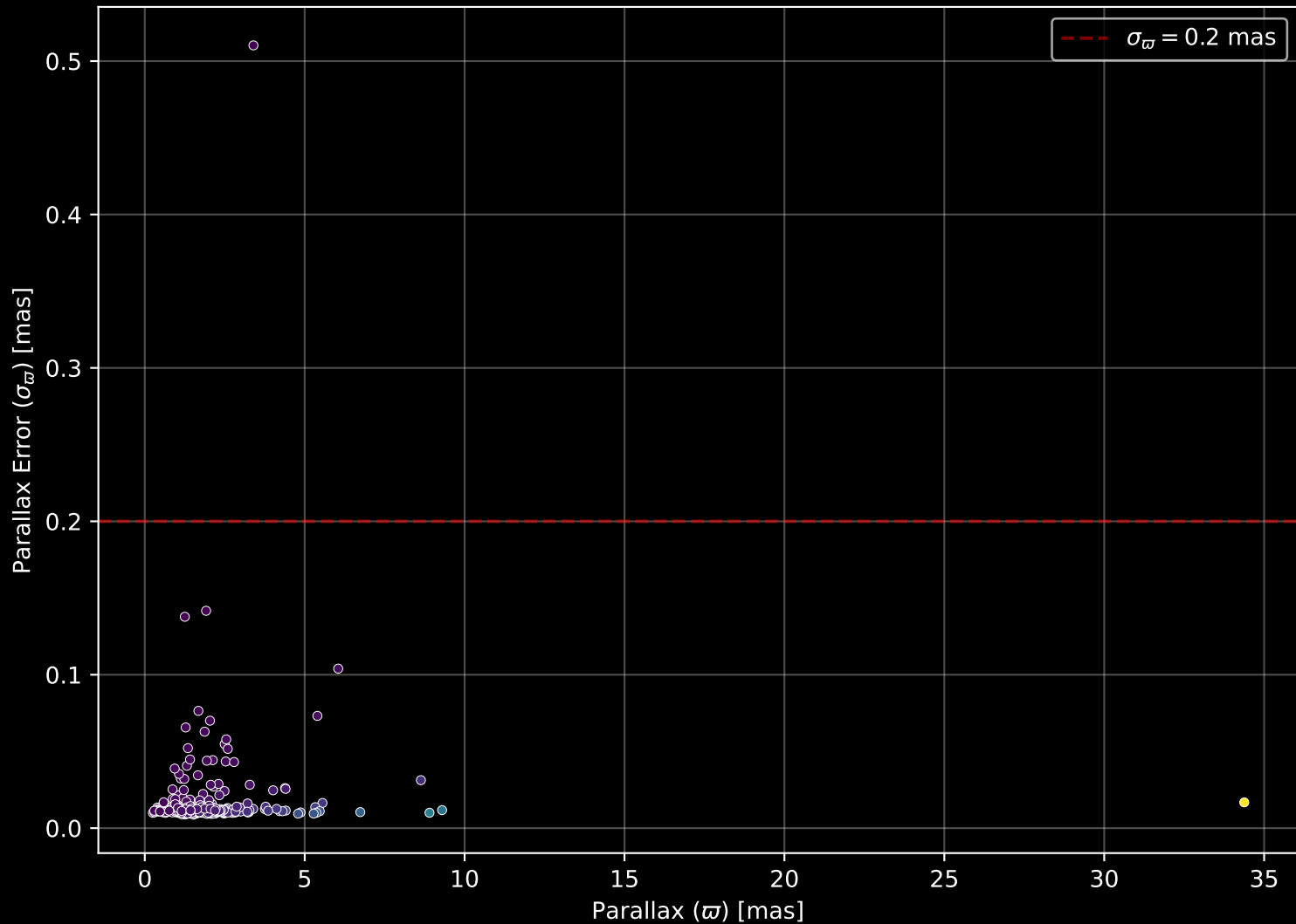
GALAH DR4 Field: [150] Parallax Quality (n= 296)
