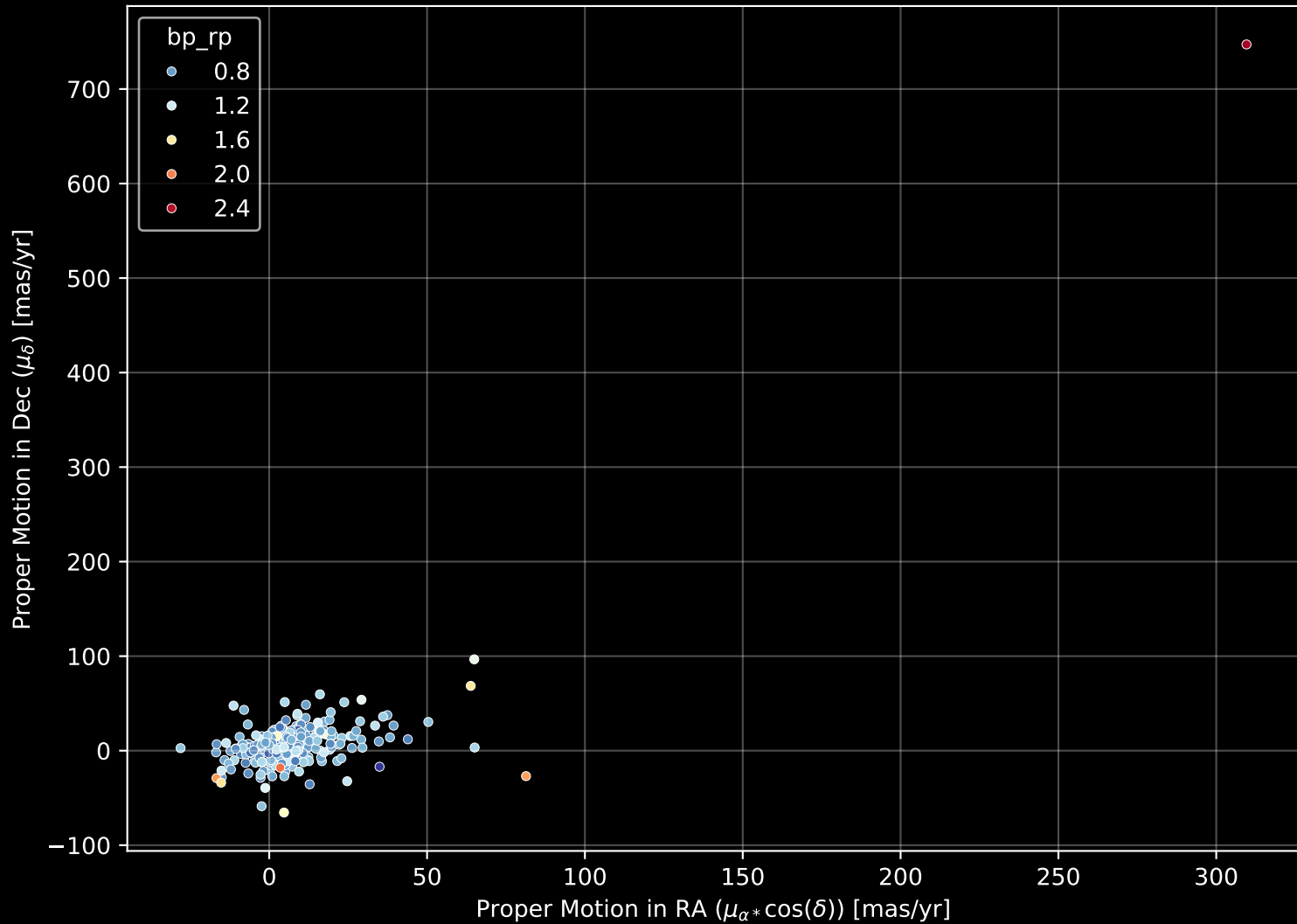
GALAH DR4 Field: [150] Proper Motion Diagram (n= 296)
