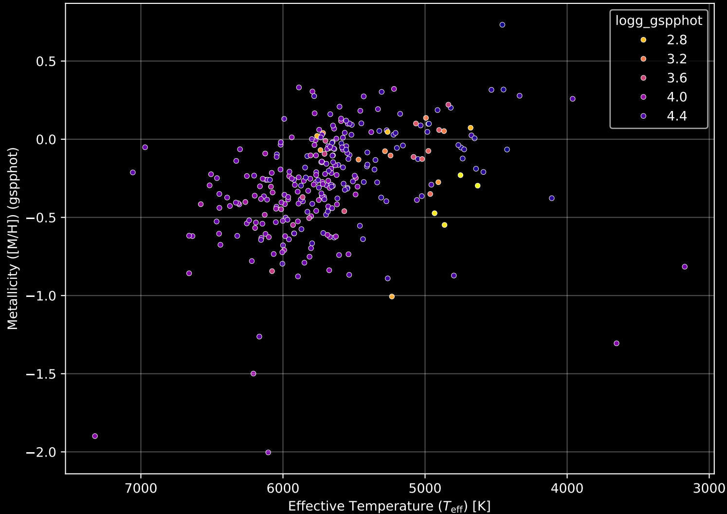
GALAH DR4 Field: [150] Stellar Population Parameters (n= 296)
